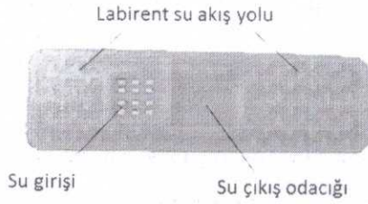
Şekil 1. SERTSAN Damla Sulama Borularında (2.2 L/h anma debili) kullanılan yassı damlaticının genel görünüşü
