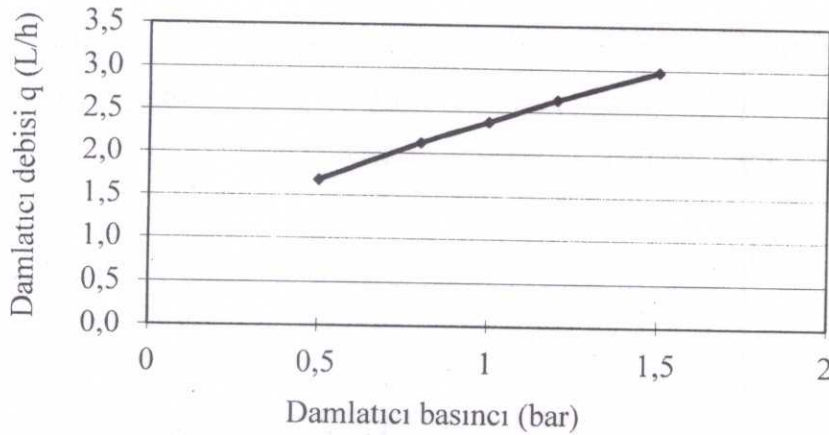
Şekil 2. SERTSAN Model Damla Sulama Boruları (2.2 L/h anma debili)'nin yassı damlatıcılarına ait basınç-debi ilişkisi
