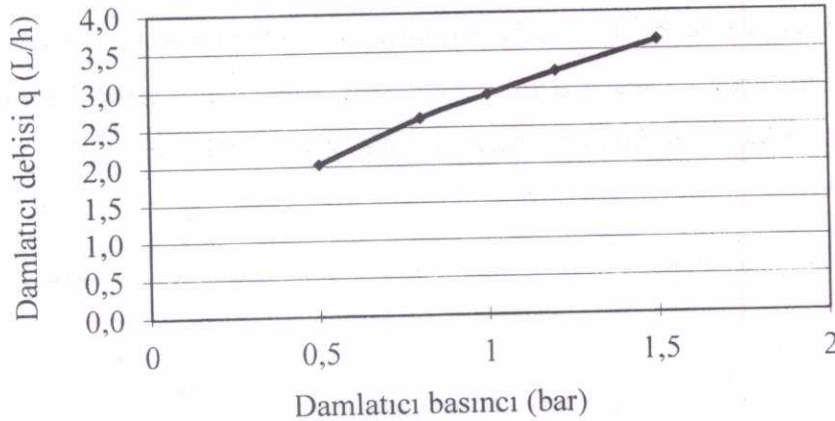
Şekil 2. SERTSAN Model Damla Sulama Boruları (2.8 L/h anma debili)'nin yassı damlaticılarına ait basınç-debi ilişkisi
