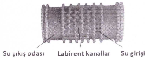
Şekil 1. SERTSAN damla sulama borularında (2.0 L/h anma debili) kullanılan silindirik damlatıcının genel görünüşü
