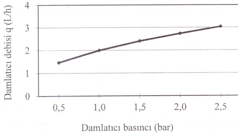
Şekil 2. SERTSAN damla sulama boruları (2.0 L/h anma debili)'nin damlatıcılarına ait basınç-debi ilişkisi
